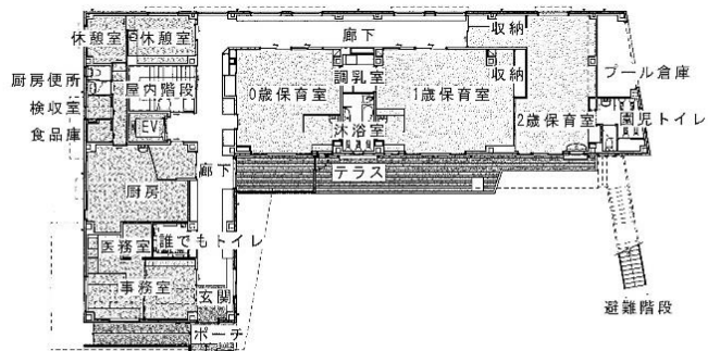
1階平面図
